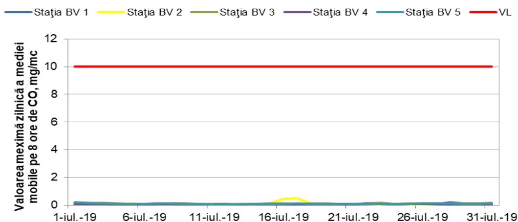
Figura 1.1.2.5.1. Evoluția maximelor zilnice ale mediei mobile de CO în luna iulie
