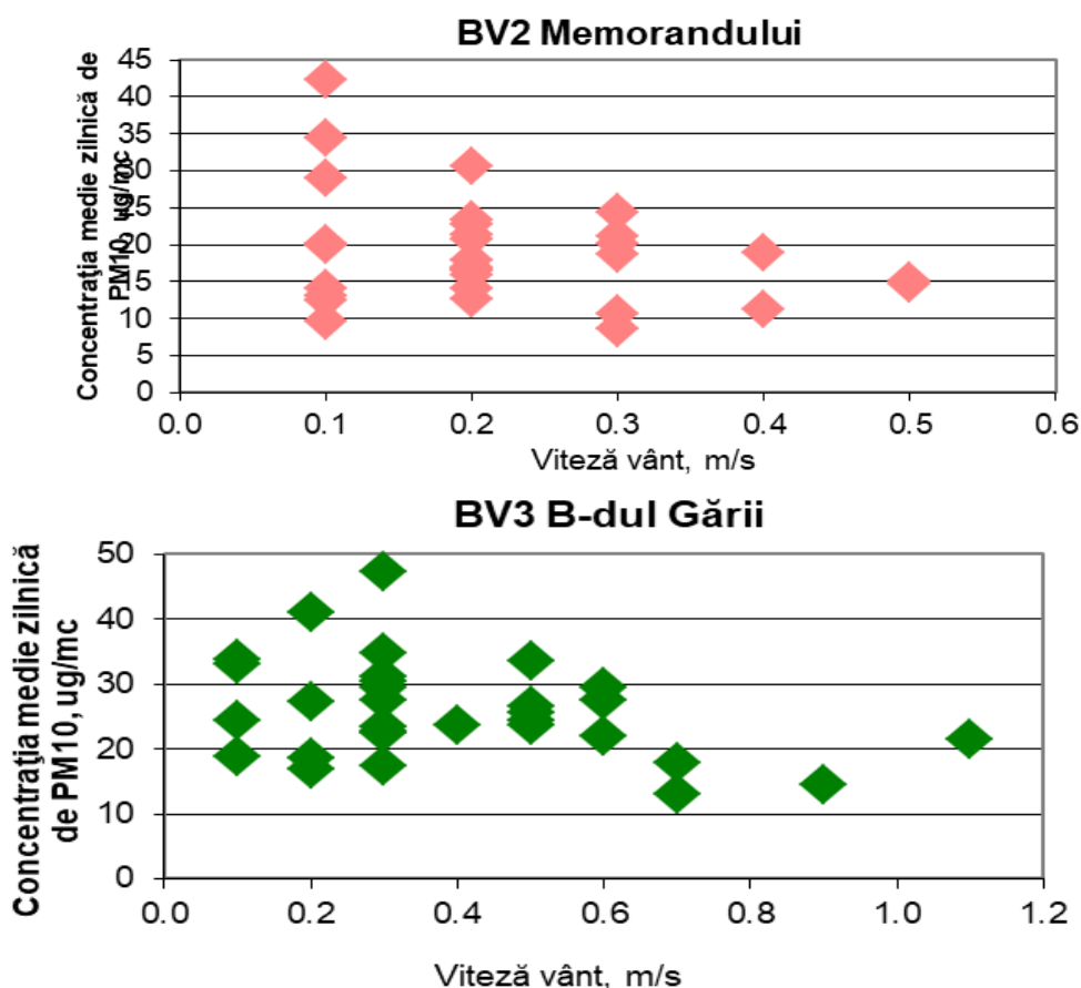
Figura 1.1.2.4.2. Evoluția mediilor zilnice de PM 10 în funcție de viteza vântului la stațiile BV2 și BV3
