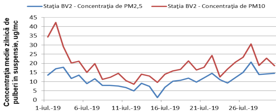
Figura 1.1.2.4.4 Evoluția mediilor zilnice de PM 2,5 și PM10 în luna iulie
