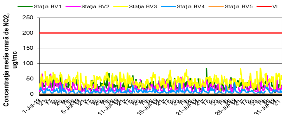
Figura 1.1.2.2.1. Evoluția mediilor orare de NO 2 în luna iulie
