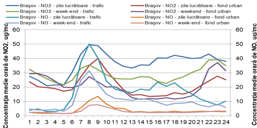
Figura 1.1.2.3. Ciclul zilnic al oxizilor de azot în timpul săptămânii
