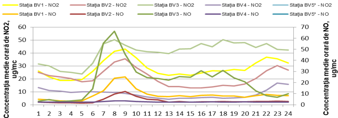
Figura 1.1.2.2. Ciclul zilnic al NO 2 și NO
